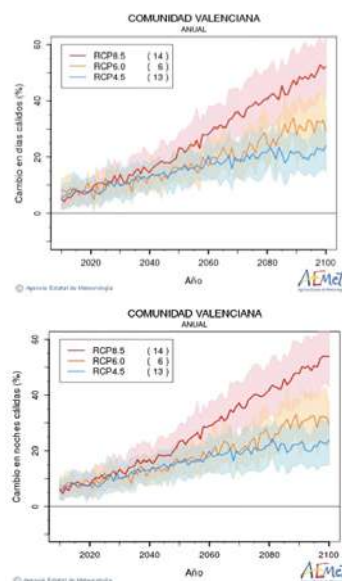
Figura 19. Cambios previstos en la duración de los días de calor y en el número de noches cálidas a 20^{\circ} \text{C} . Proyección 2000-2100 (respecto al período de referencia 1961-2000)
