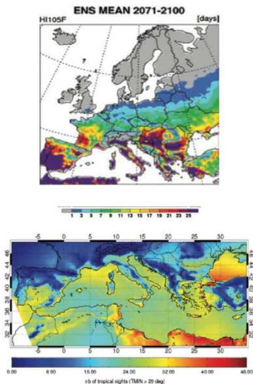
Figura 18. Cambios previstos en el número de días con temperaturas máxima > 40^{\circ} \text{C} y temperatura mínima superior a 20^{\circ} \text{C} . Proyección 2071-2100 (respecto al período de referencia 1961-90)
